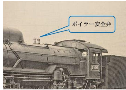
【蒸気機関車 D51 とボイラー安全弁】
